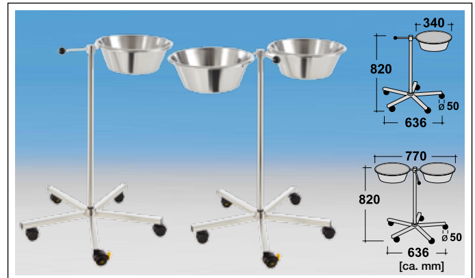
NIRO-STERI-FIX - Fußkreuz fugenfrei verschweiß Nr. LD 627 16 1 Schale, Gesamtgewicht ca. 7,5 kg € 269,- Nr. LD 627 17 2 Schalen, Gesamtgewicht ca. 8,8 kg € 329,-
