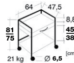
Maße CROMOSTAR
