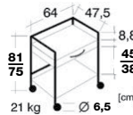
Maße QUICKSTAR
