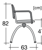
Maße System ALEXA
