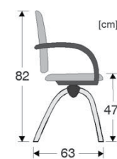
Maße System LINEA mit Sitz VISITE
