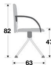
Maße in cm System ELEGANCE mit Sitz VISITE
