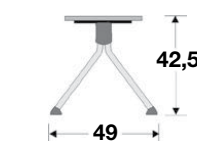
Maße in cm System ELEGANCE mit Tischplatte
